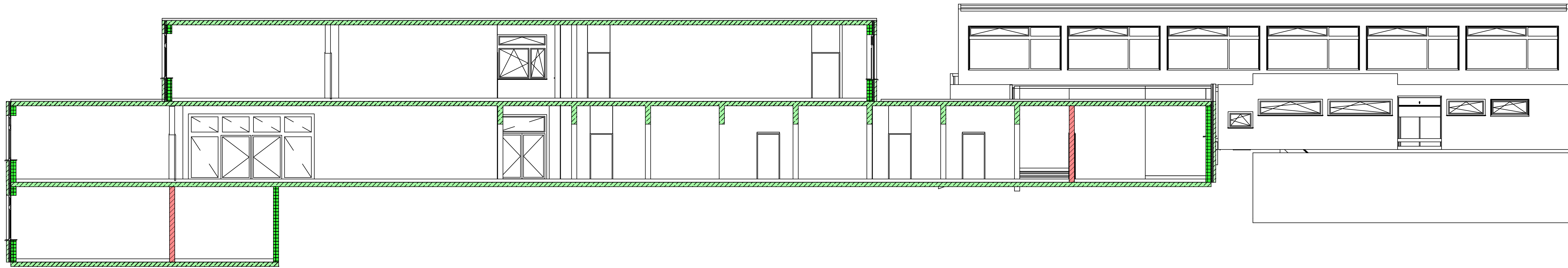
Ansicht A-A
